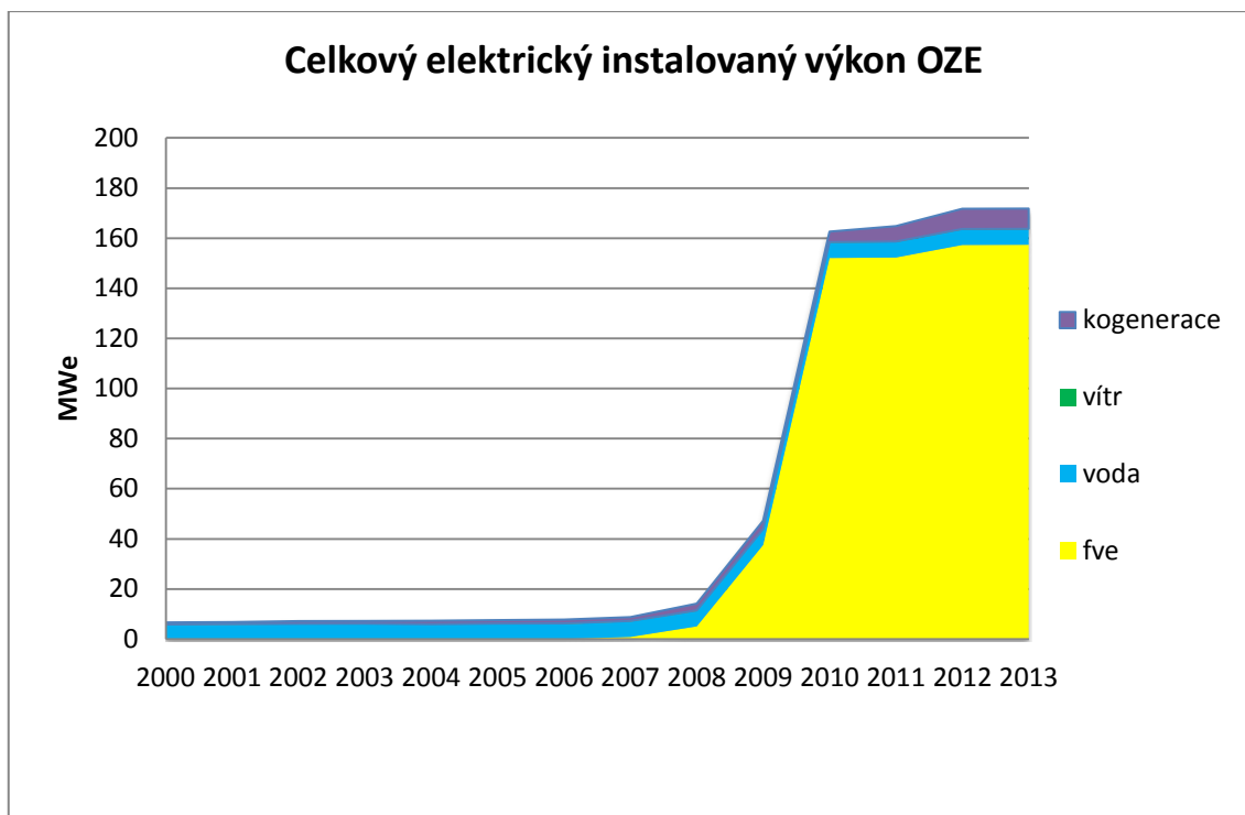
Obr. 6: Celkový instalovaný výkon OZE ve ZK (zdroj: Katalog OZE ZK, vlastní tvorba, 2014)
