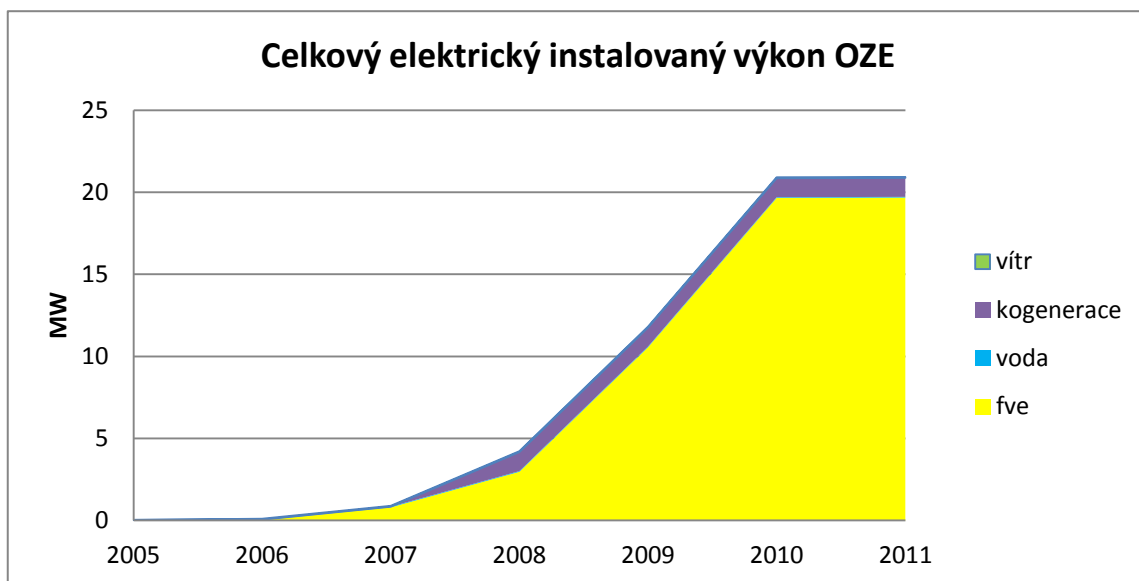
Obr. 8: Vývoj instalovaný výkonu OZE v SO ORP Uherské Hradiště v letech 2005 -2014 (zdroj: ERÚ, vlastní tvorba, 2014)
