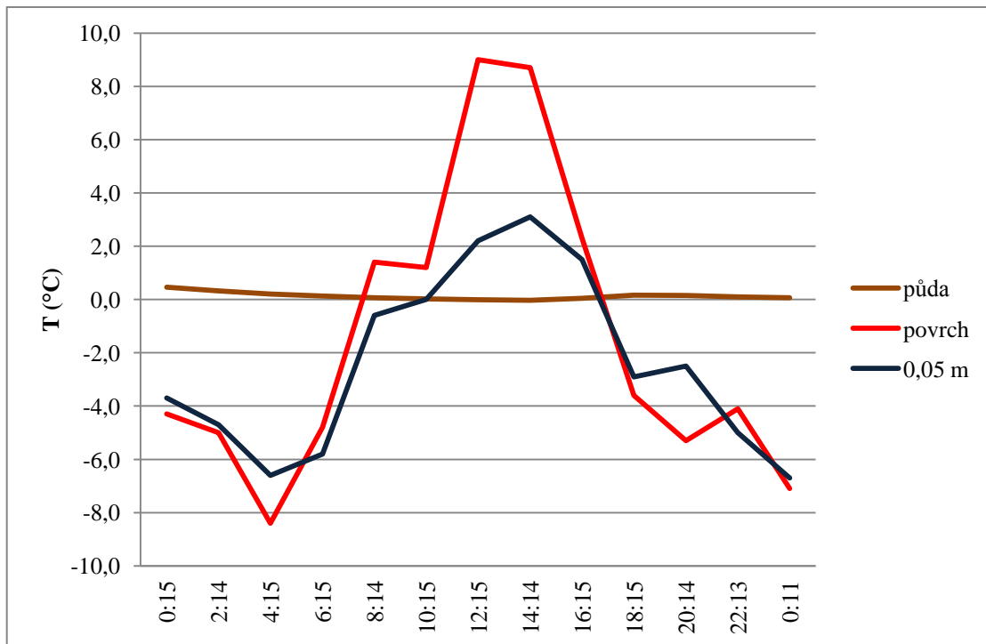
Obr. 20: Režim teploty půdy, povrchové teploty a teploty vzduchu 0,05 m nad aktivním povrchem na experimentální ploše Letiště Olomouc 6. 3. 2012
