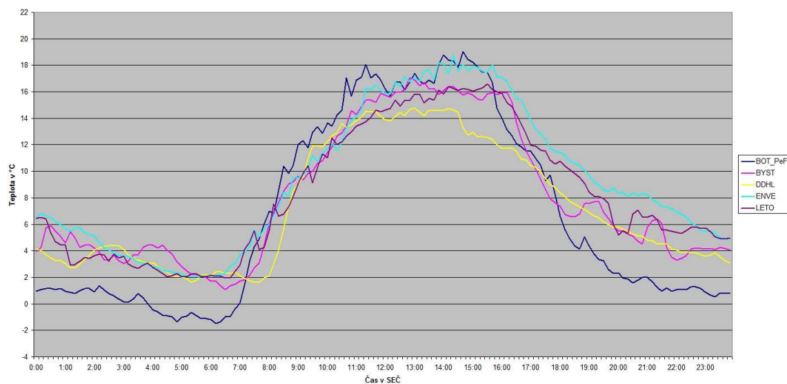
Obr.23: Denní chod teploty vzduchu na vybraných stanicích 11. 10. 2010 (Zdroj: MESSO Olomouc)
