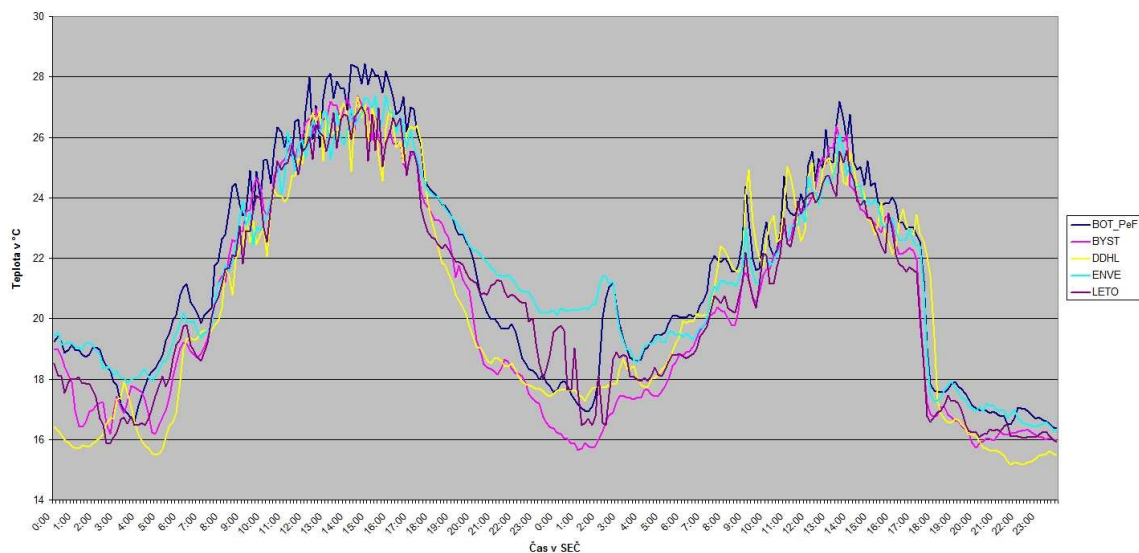
Obr.31: Denní chod teploty vzduchu na vybraných stanicích 7. 6. a 8. 6. 2010 (Zdroj: MESSO Olomouc)
