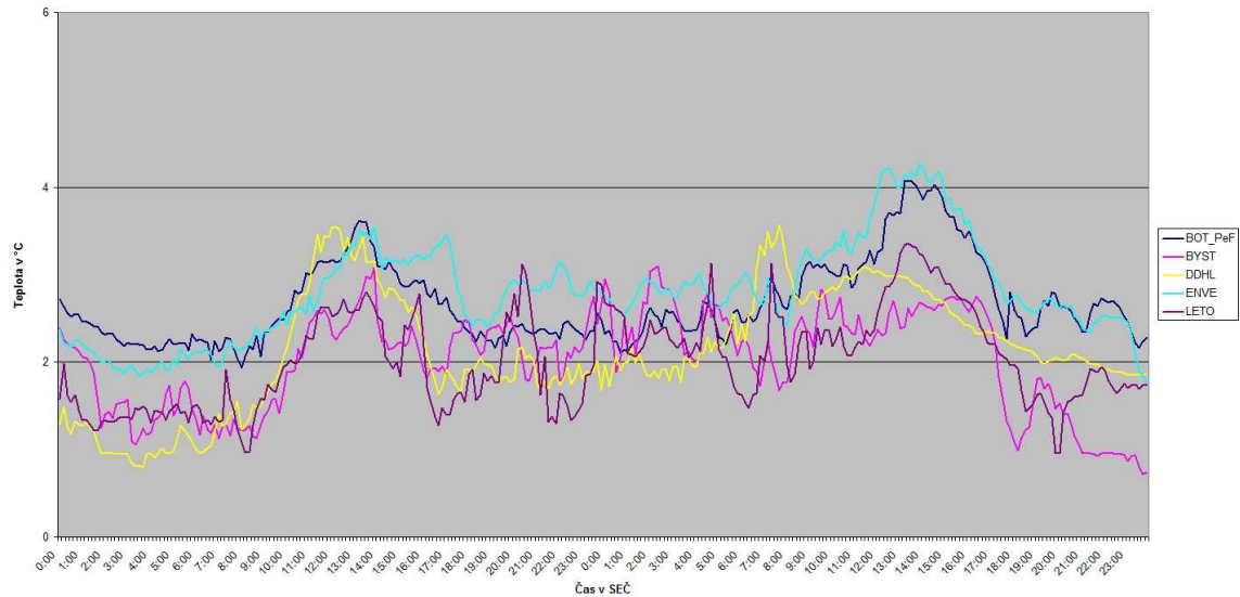
Obr.28: Denní chod teploty vzduchu na vybraných stanicích 9 .1. a 10 .1. 2010 (Zdroj: MESSO Olomouc)
