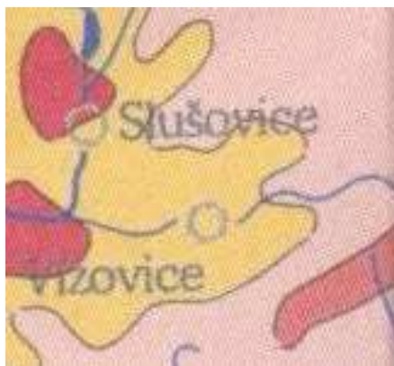
Obr. 2: Schéma druhů půd (podle Tomáška)
