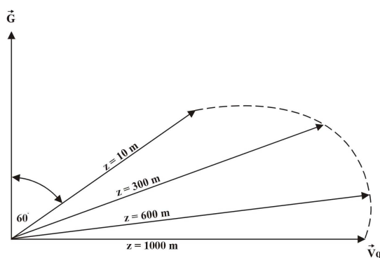
Obr. 29: Ekmanova spirála
