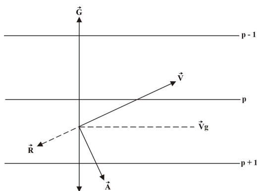
Obr. 28: Rovnoměrný přímočarý pohyb bez tření
