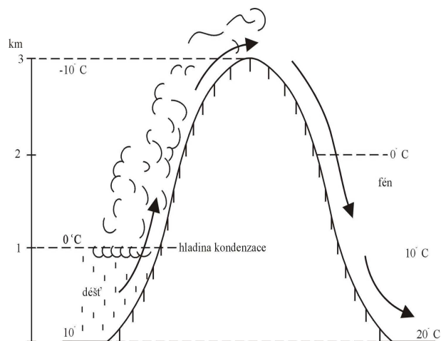
Obr. 38: Vznik fénu (vlastní zpracování)
