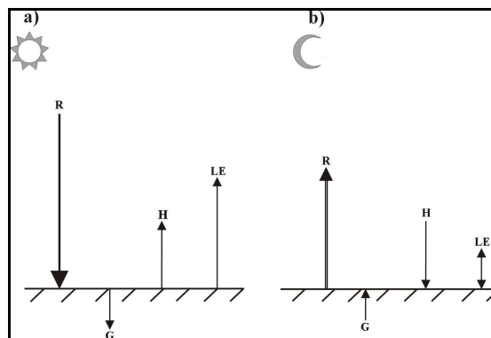
Obr. 17: Složky energetické bilance zemského povrchu v období a) pozitivní a b) negativní energetické bilance ( R - radiční bilance, G - tok tepla do podloží aktivního povrchu, H - turbulentní tok tepla, LE - latentní tok tepla)
