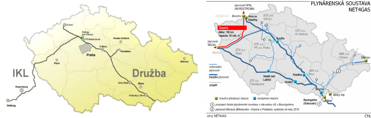
Obr. 7.8: Ropovody a plynovod nadzemí ČR
